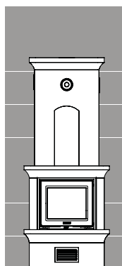
Brandvägg 1140 mm K10 mot rakvägg.
