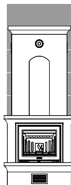
Brandvägg 900 mm K20 mot rakvägg.
