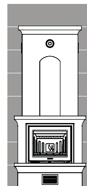
Brandvägg 1140 mm K20 mot rakvägg.
