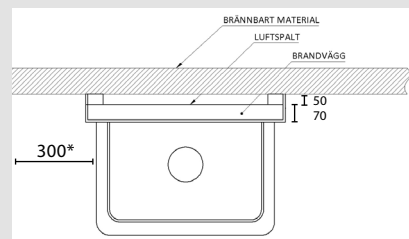
Brandvägg 900 mm K20 mot rakvägg.
