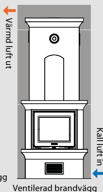
Brandvägg 900 mm K10 mot rakvägg.
